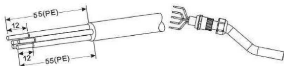
Рисунок 18 Обработка кабеля
