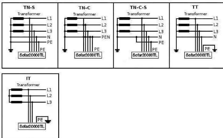
Компоненты Рисунок 2 Варианты инвертора топологии сети
