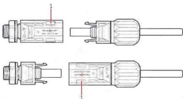
Рисунок 32 Подключение кабелей входной мощности постоянного тока (DC)
