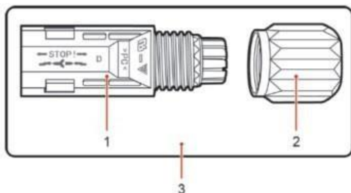
Рисунок 29 Состав отрицательного коннектора
