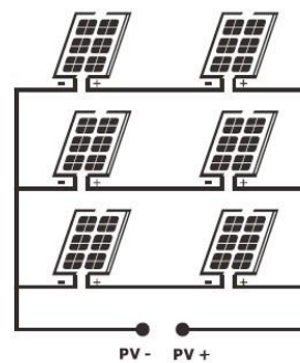
MPPT-60A (2кВт)
